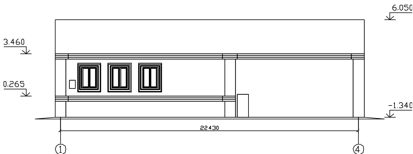
Фасад 1-4 после реконструкции M1:100
