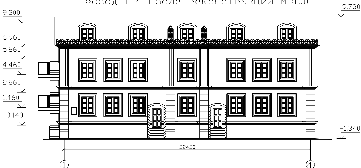
Фасад 1-4 после реконструкции M1:100
