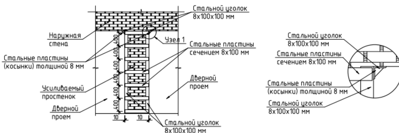
Рис. 10. Пример оформления схемы усиления столба стальной обоймой (сечение по усиленному элементу условно не показано).
