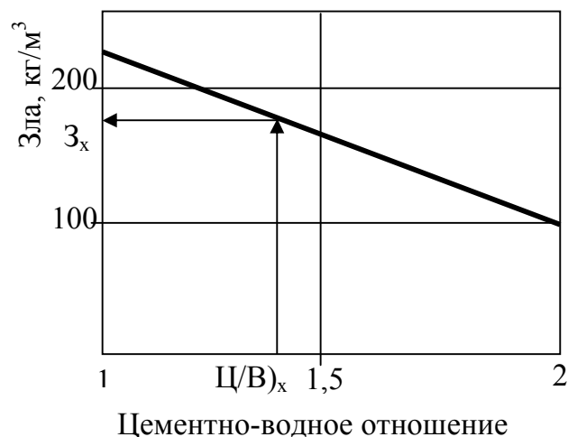
Рис. 2. Зависимость оптимального расхода золы от Ц/В
