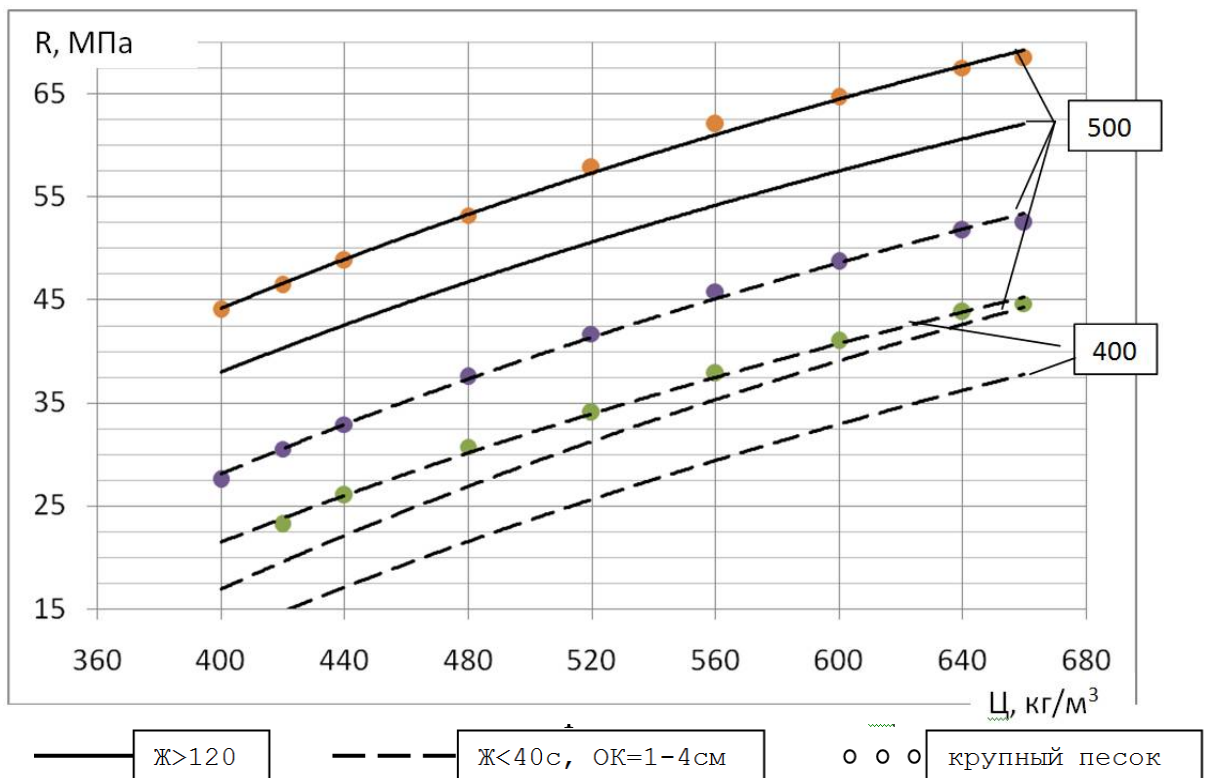
Рис.1. Изменение прочности бетона от Ц/В
