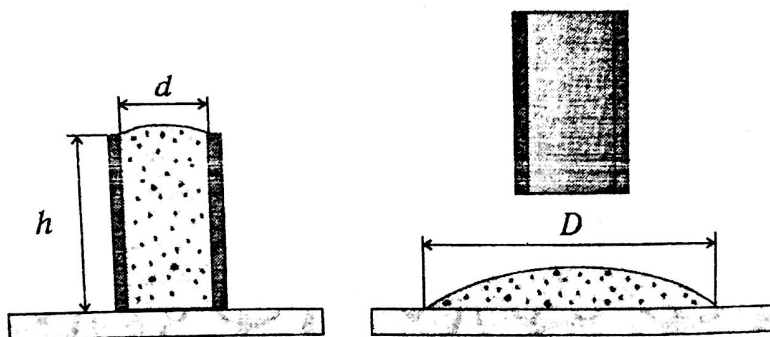
Рис. 1. Цилиндрический вискозиметр
