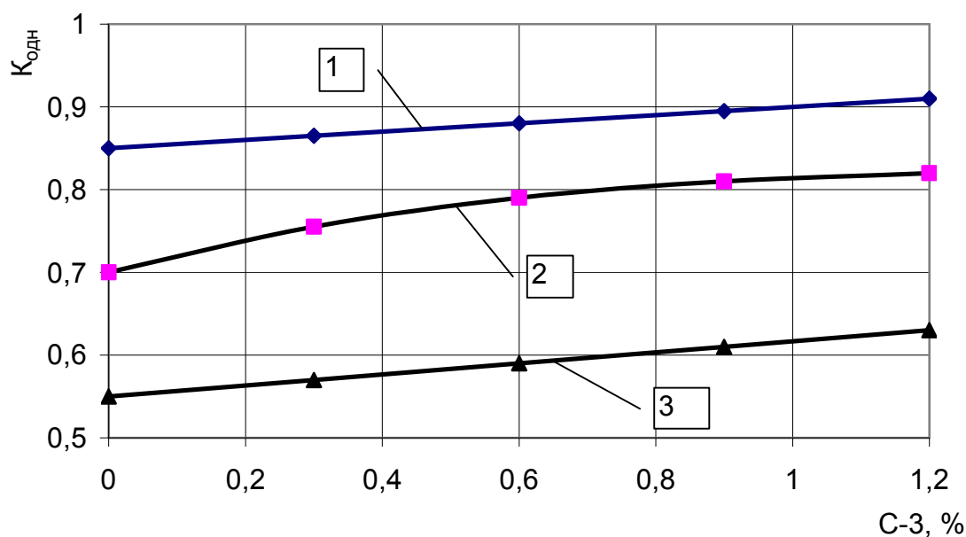
Рис.1. Зависимость коэффициента однородности бетонных смесей от дозировки суперпластификатора С- 3:
