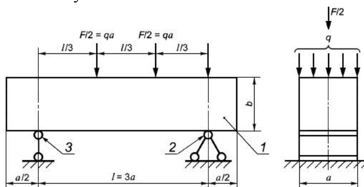
Рис. 3. Схема испытания на растяжение при изгибе
