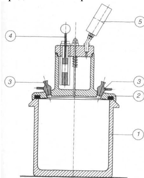
Рис.4. Схематическое представление прибора для определения объема воздухововлечения бетонной смеси:
