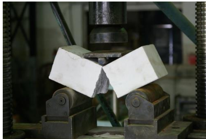
Испытание силикатного кирпича на изгиб
