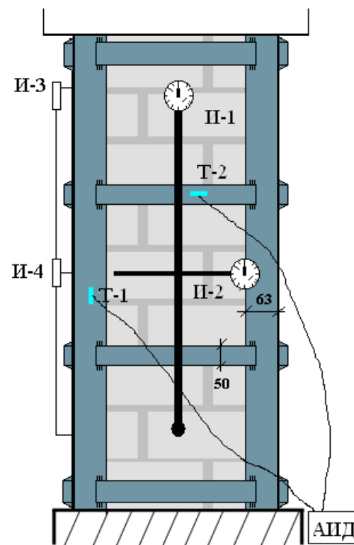
Рис. 1. Расстановка измерительного оборудования
